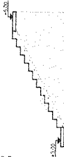
Escaleras de Hormigón Formadora de reparación Suelo contrapunto Vereda de H con junta
