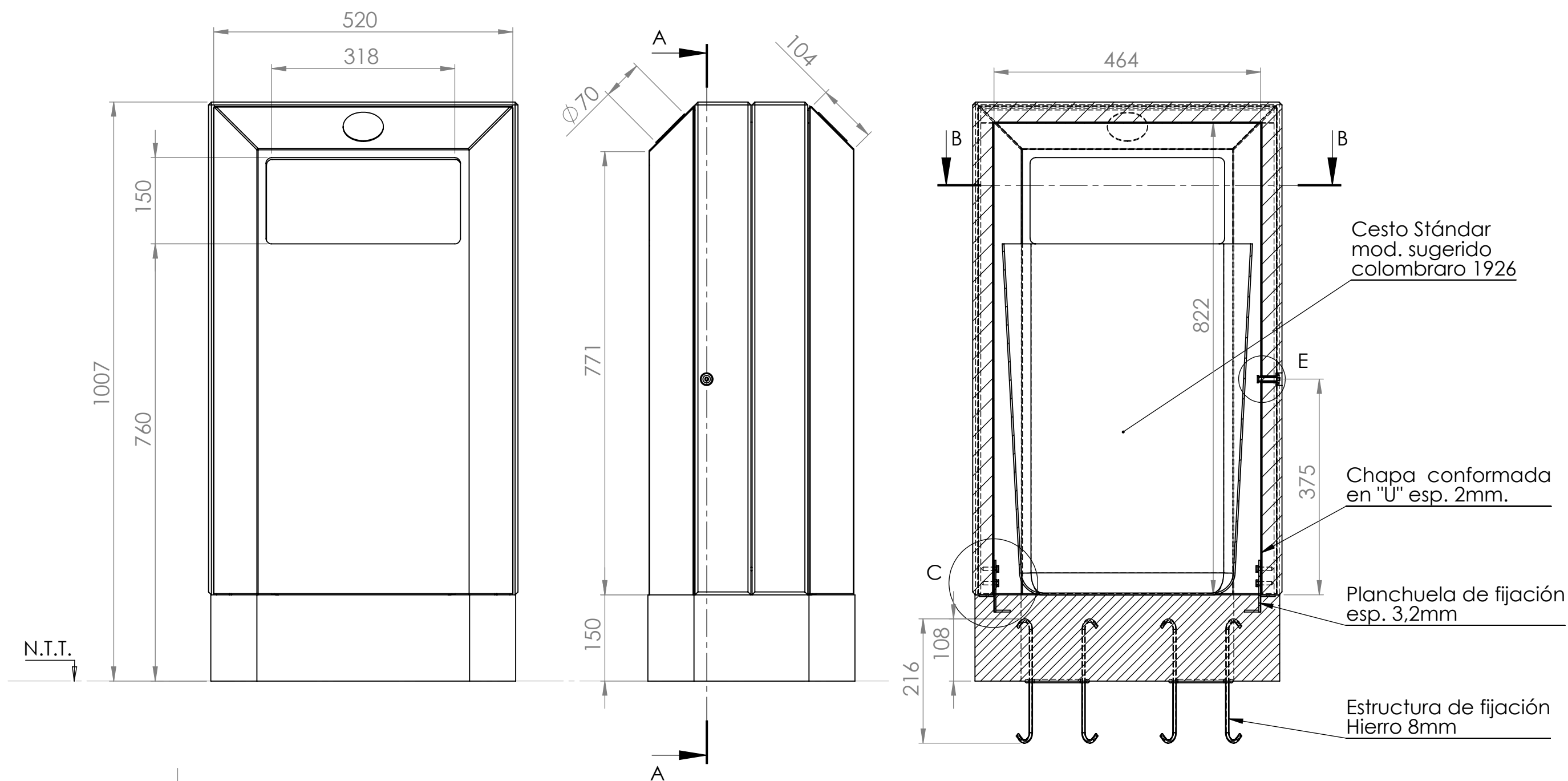
SECCIÓN A-A
